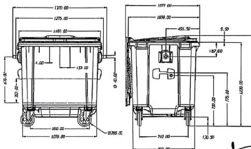
Gráfico 2. Dimensiones y estructura de los contenedores de 1.100 litros.
